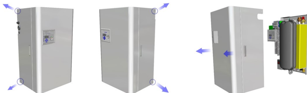
Slika 5. Otvaranje kotla (demontaža prednjeg omotača kotla)
