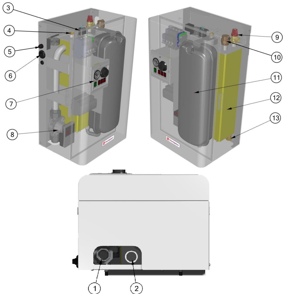
Slika 2. Komponente kotla
